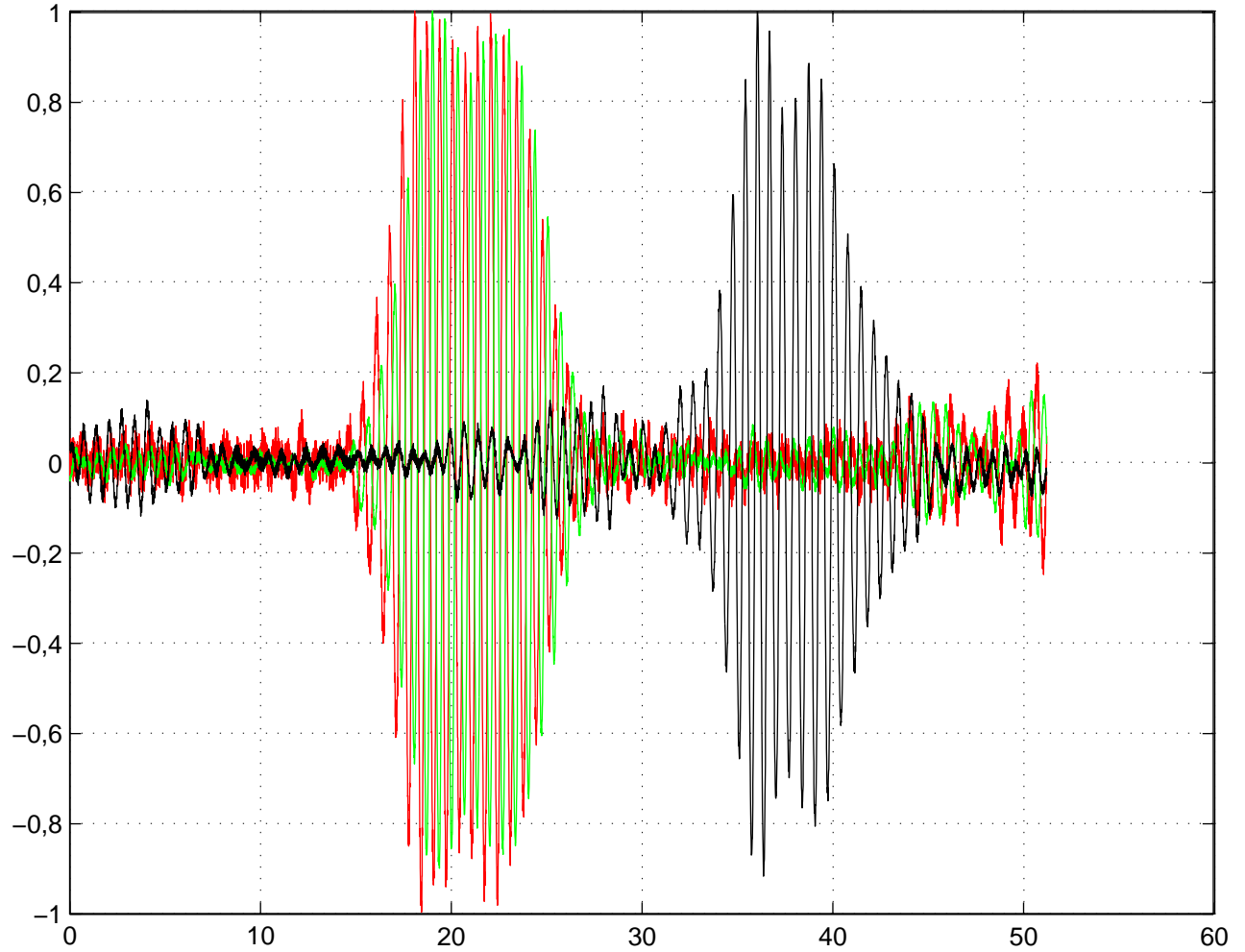
13.00 datos del sensor de oleaje para 1,5 Hercios
