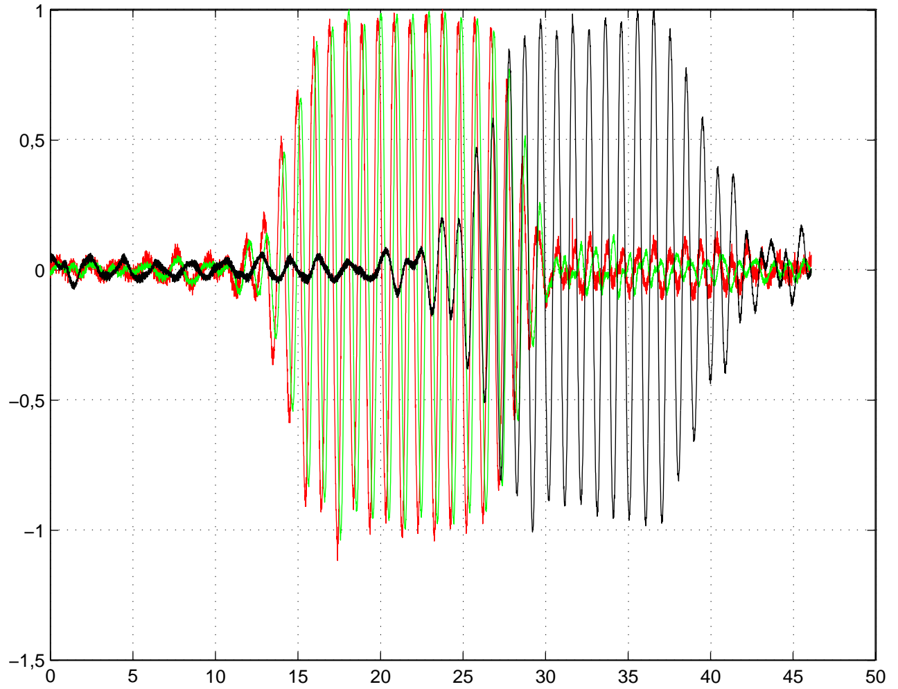
13.00 datos del sensor de oleaje para 1,0 Hercios
