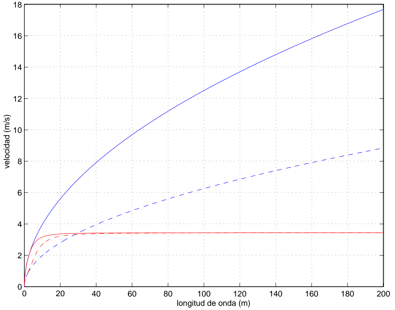
velocidad frente a longitud de onda para profundidad de aguas inf. y para h=1,2 metros
