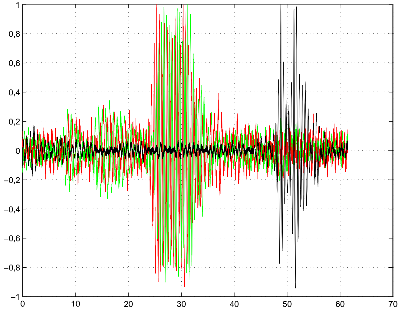
13.00 datos del sensor de oleaje para 2,0 Hercios
